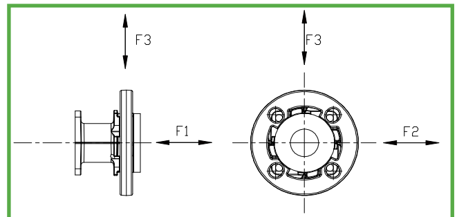
Figure 12 Charges de Buses sur les Brides
