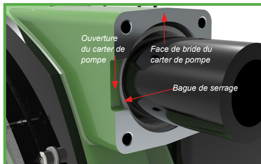
Figure 8 Anneau de serrage inséré
