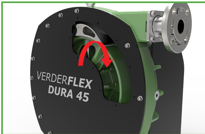
Figure 10 Remplissage de la Pompe avec le Lubrifiant
