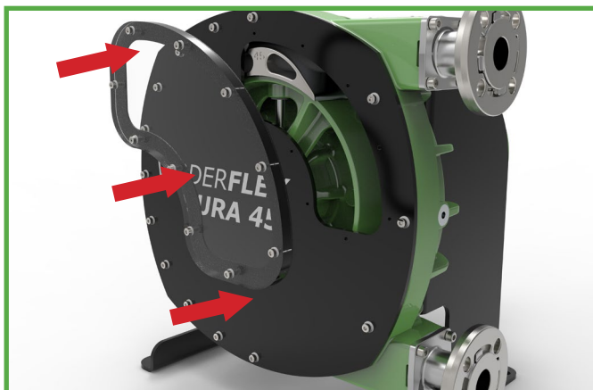
Figure 11 Installation de la Fenêtre d'Inspection
